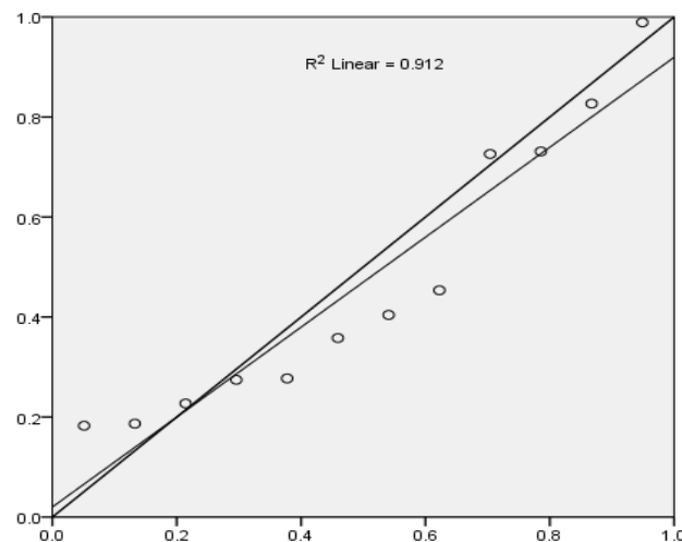
Gambar 3. Grafik regresi linier
