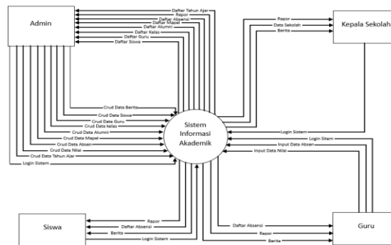
Gambar 2. Diagram Konteks
