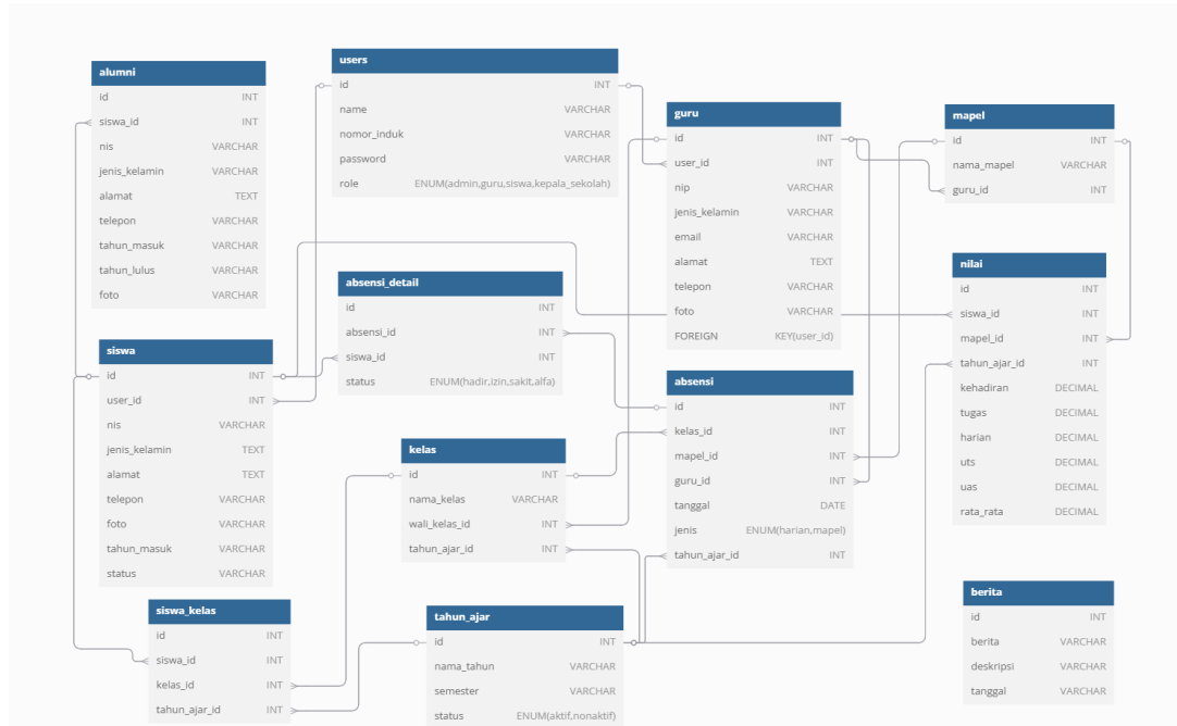
Gambar 9. Relasi Database
